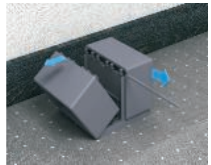
Gehäuse T4B und T12L öffnen Achse herauschieben und Gehäusehälften abklappen.
