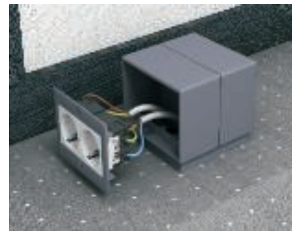
Montage Modul 45-Geräte in T4B und T12L Vor dem Leitungsanschluss das Modul 45-Gerät in die Abdeckplatte einrasten.
