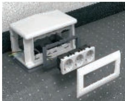
Installation Modul 45-Geräte in T4L und T8NL Leitungsöffnungen in Gerätebecher Telitank T4L vorbereiten und in Gehäuse einrasten. Modul 45-Gerät vor Leitungsanschluss in Abdeckplatte einrasten.
