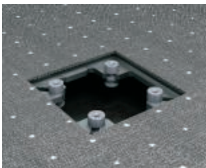
Einsetzmutter in blind abgedeckten DAT-Öffnungen Einsetzmutter entsprechend der benötigten Höhe in Systemöffnung DAT einschieben.
